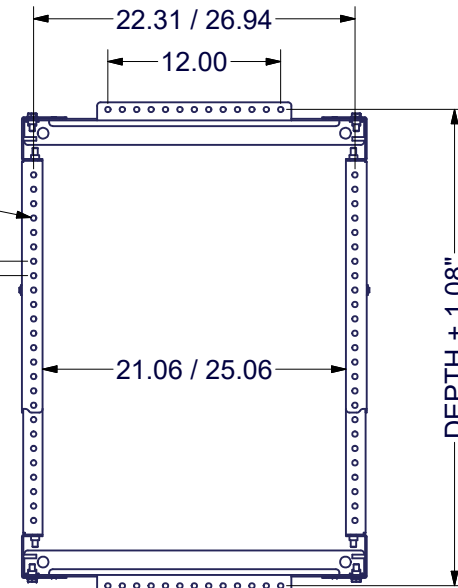
VIEW A-A
